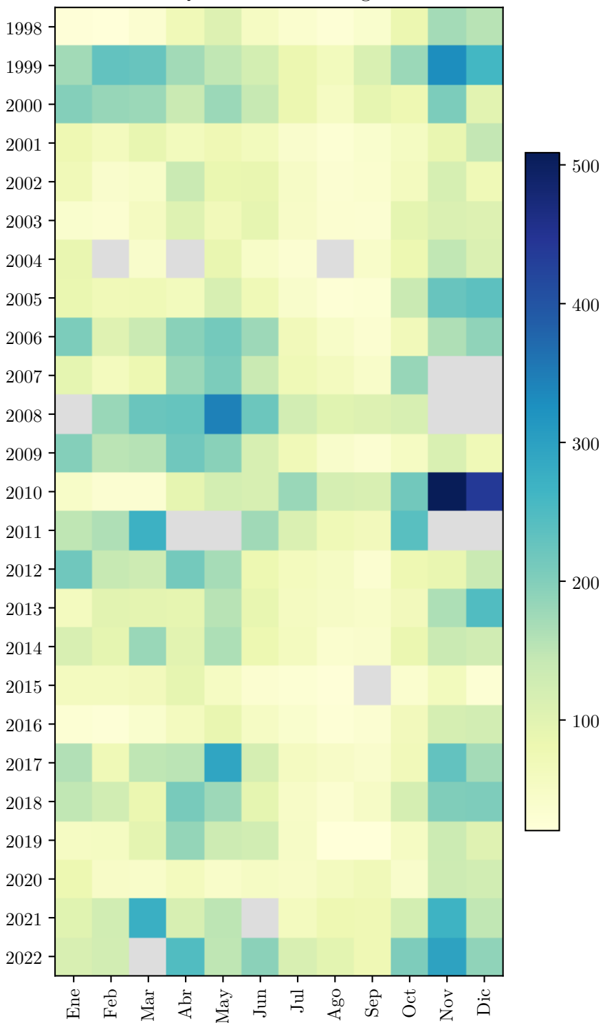
Q: caudal en Cartago
